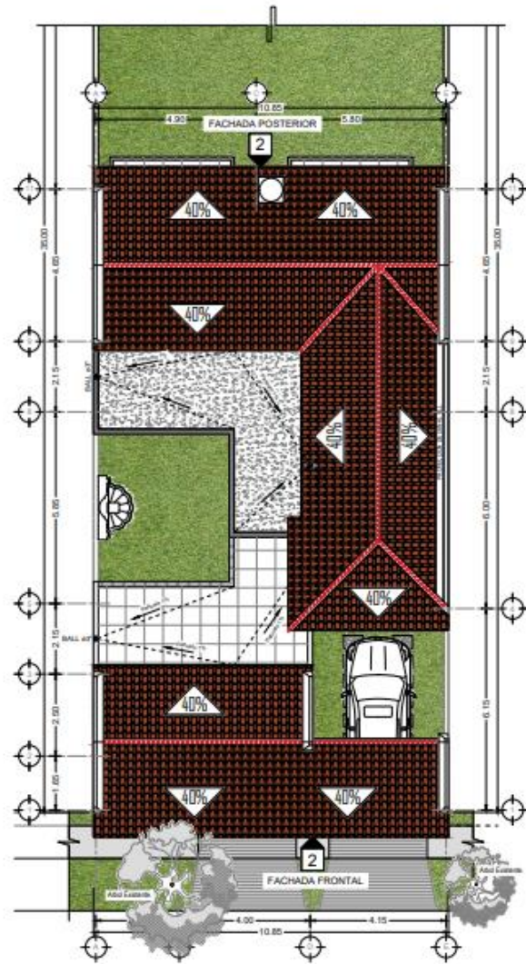
1 Planta de Techos Villa Chateau ESCALA 1:100
