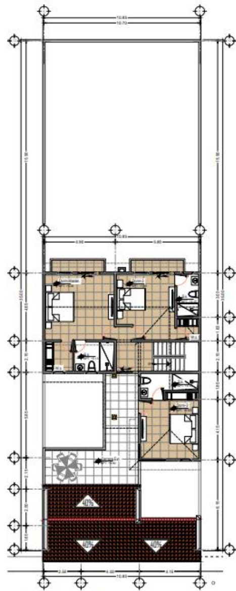
1 Planta Alta - Amoblada Villa Chateau ESCALA 1:125
