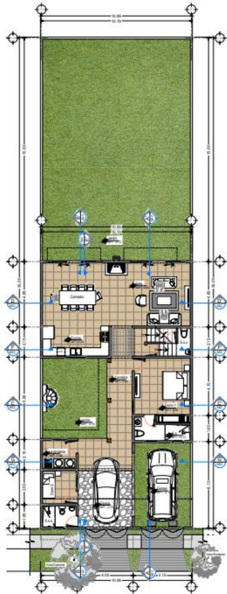
1 Planta Baja - Amoblada Villa Chateau ESCALA 1:125
