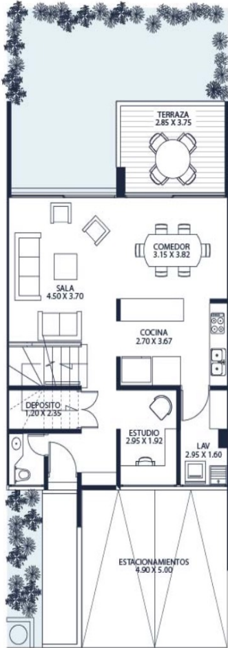
Nivel 01
