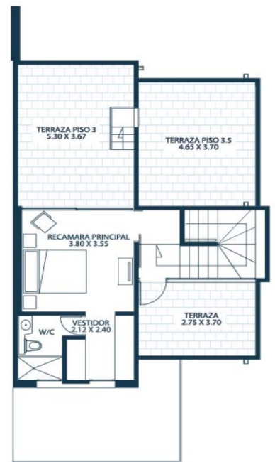
Nivel 03
