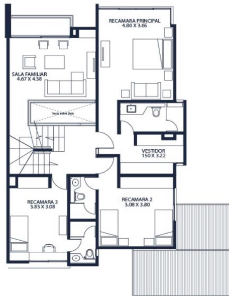
Nivel 02
