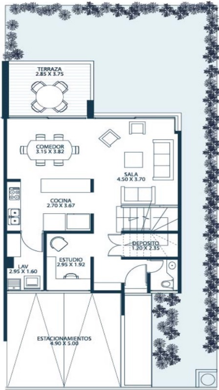
Nivel 01
