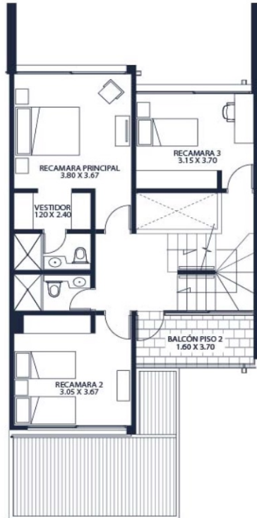
Nivel 02
