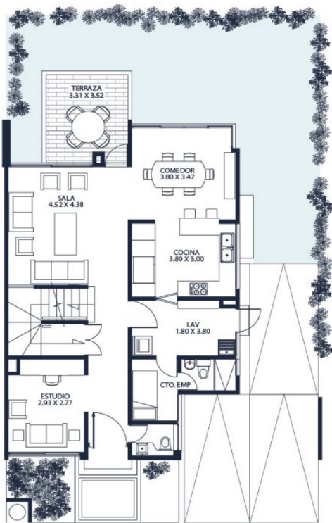
Nivel 01
