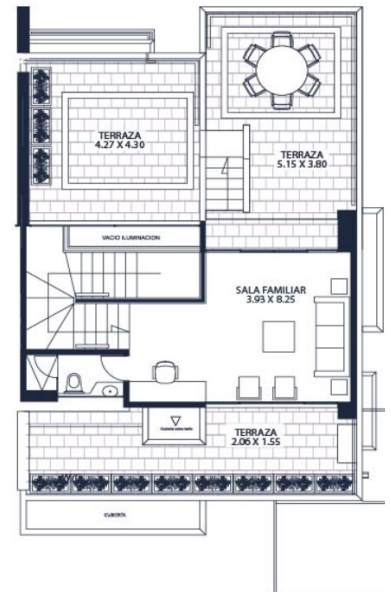
Nivel 03
