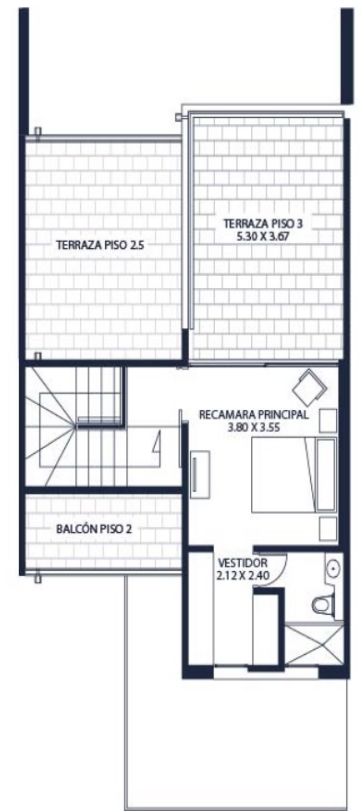
Nivel 03
