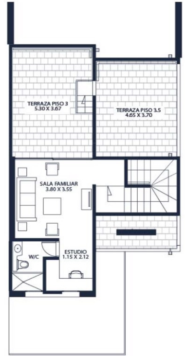
Nivel 03
