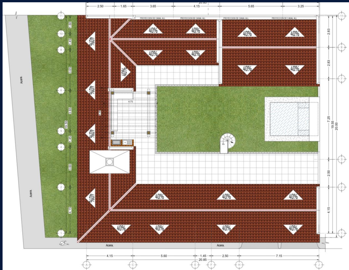
1 Planta de Techos Casa Opera Lote 32-33
