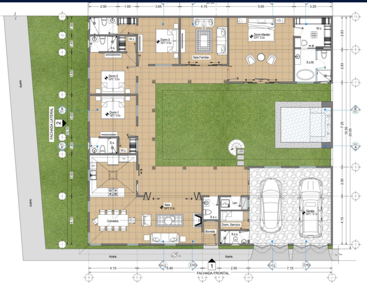
1 Planta Baja - Amoblada Casa Opera Lote 32-33
