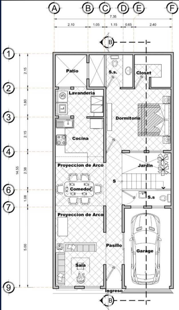
PLANTA BAJA AMUEBLADA Escala Grafica 1:50 ESCALA 1/50
