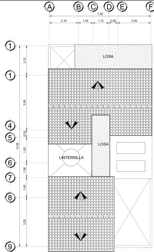
PLANTA DE TECHOS Escala Grafica 1:50 ESCALA 1/50
