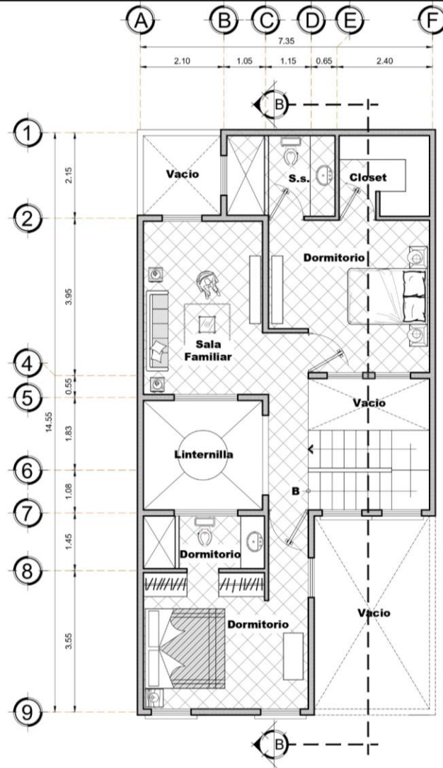
PLANTA ALTA AMUEBLADA Escala Grafica 1:50 ESCALA 1/50
