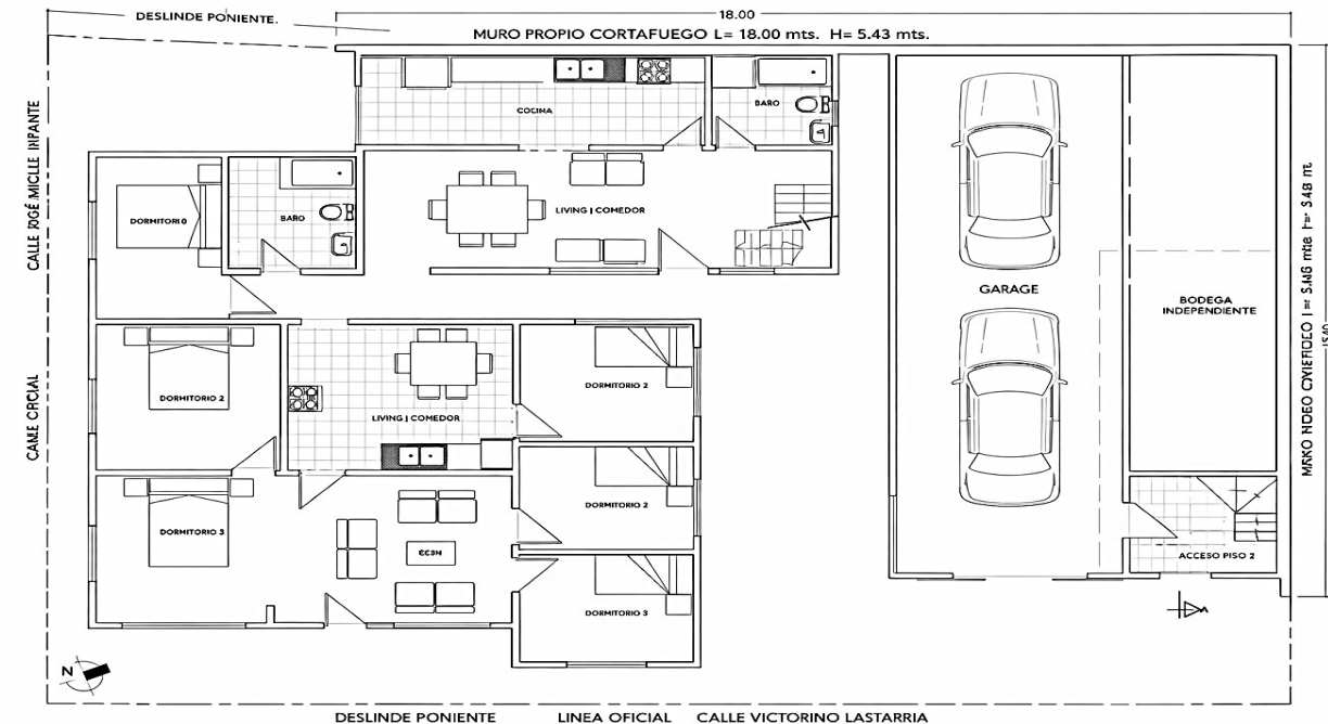
PLANTA ARQUITECTURA 1ER PISO ESCALA 1:50
