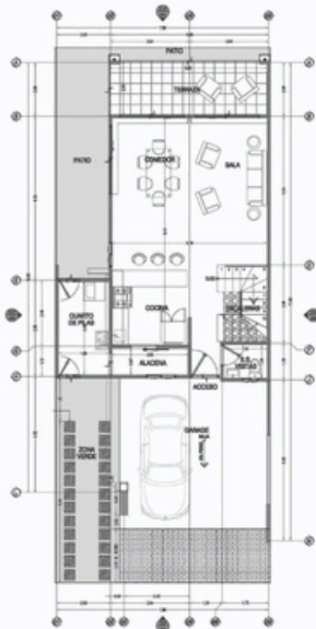
PLANTA DE DISTRIBUCIÓN ARQUITECTÓNICA PRIMER NIVEL - CASA TIPO 2C 1:50
