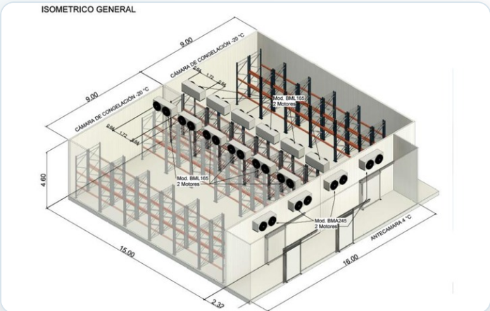
ISOMÉTRICO GENERAL — CUARTO 4 Y 5 (15 x 9 x 4.6-6 M)
