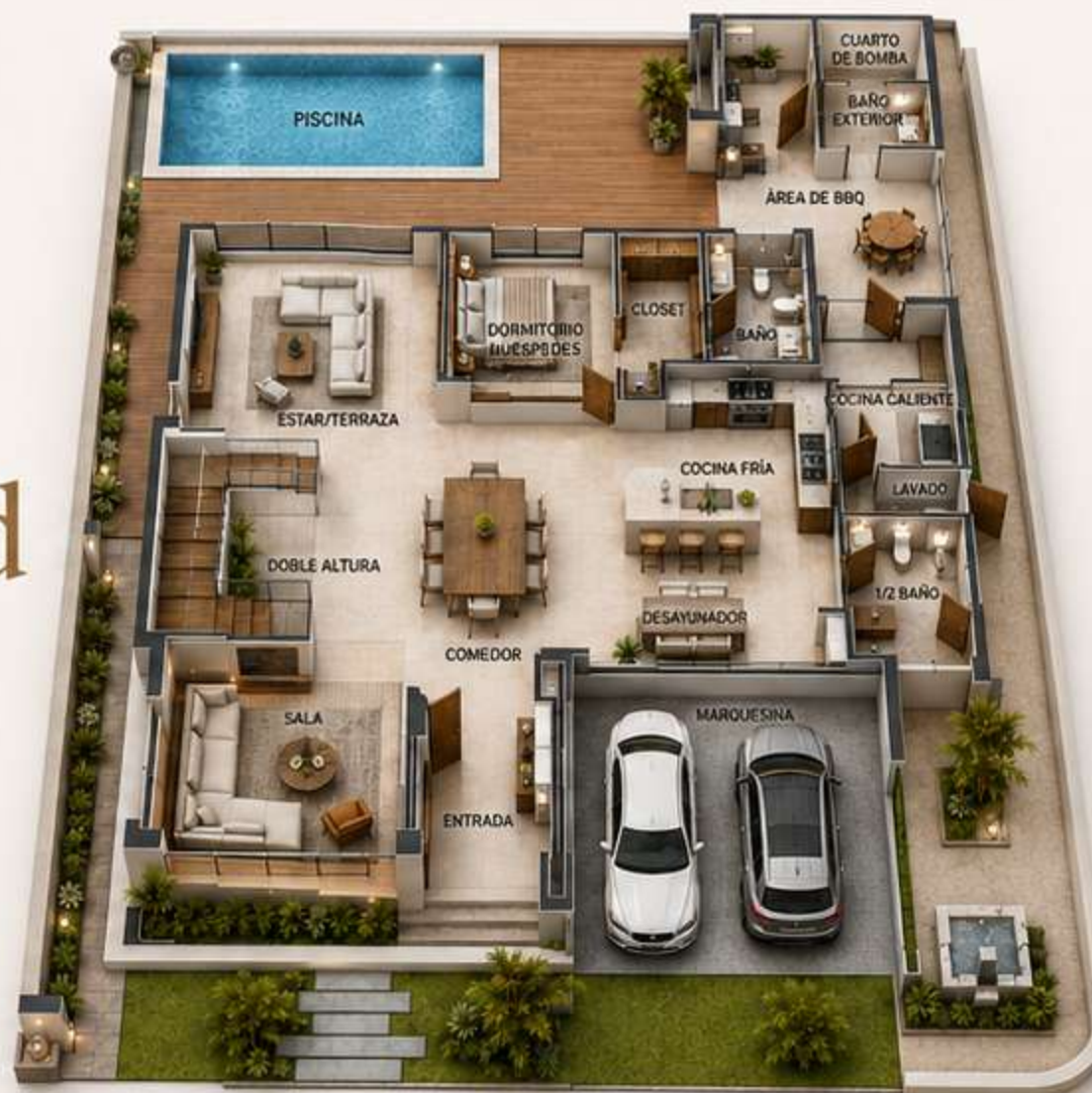
PLANTA BAJA
