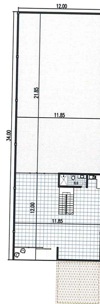
PISO 2 Oficina Principal 145,80 mts 2 (Baño y Cocineta)
