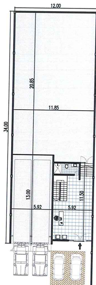
PLANTA BAJA Área de descarga 72,90 mts 2 Recepción 72,90 mts 2 - (baño) Bodega Principal 267,29 mts 2
