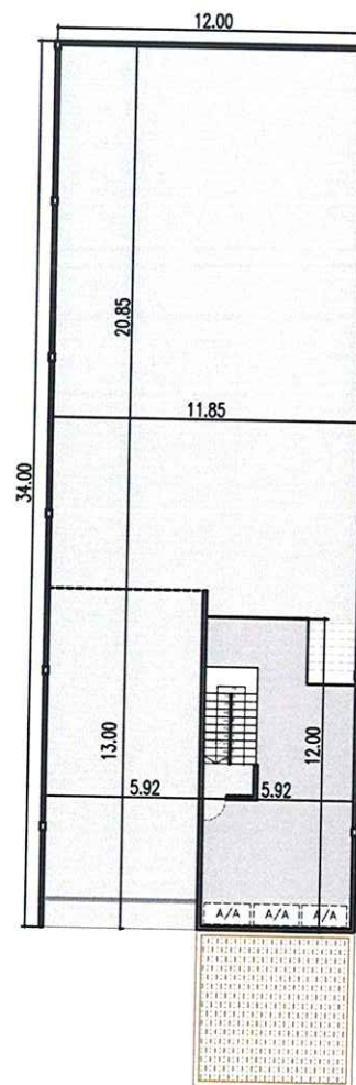
PISO 1 Depósito 72,90 mts 2
