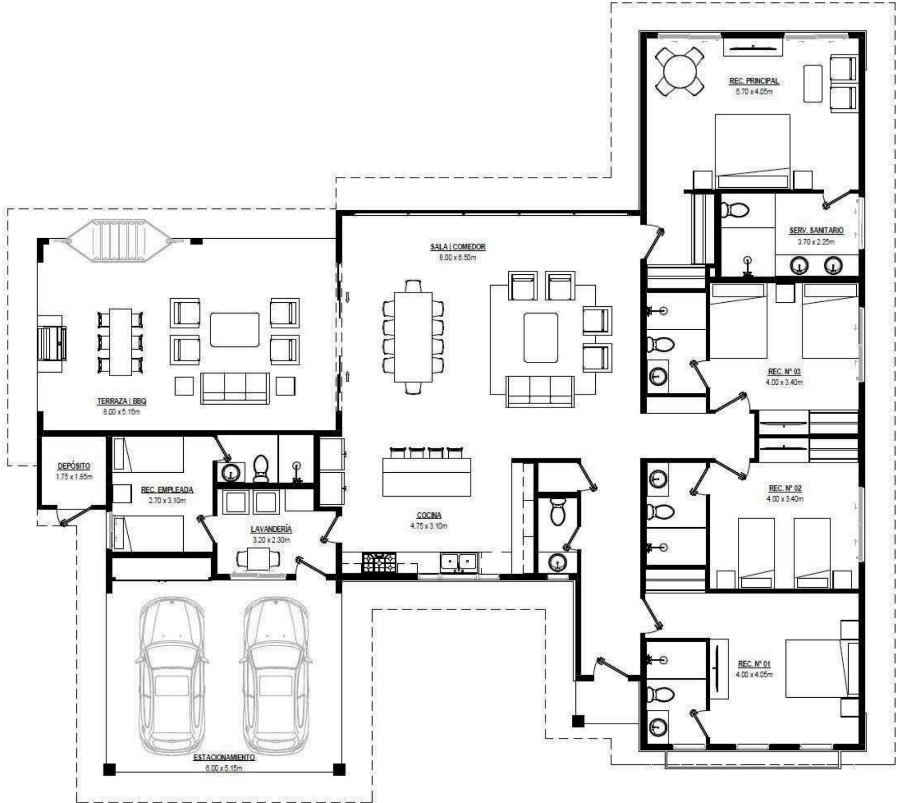
PLANTA ARQUITECTÓNICA NIVEL 000 ESCALA 1 : 100
